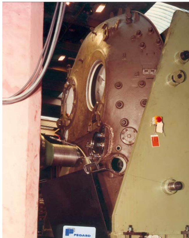
Preciram 4 – changeur d'outils à chaîne – pick-up avec appareils à fraiser
